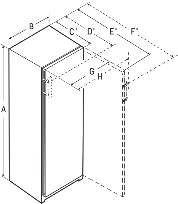
Fig. 3 A = altura del electrodoméstico incluidas patas/ruedas/bisagra B = anchura del electrodoméstico sin tirador C = profundidad del electrodoméstico sin tirador D = profundidad del electrodoméstico con tirador E = profundidad del electrodoméstico con la puerta abierta sin tirador F = profundidad del electrodoméstico con la puerta abierta con tirador G = anchura del electrodoméstico con la puerta abierta sin tirador H = anchura del electrodoméstico con la puerta abierta con tirador
